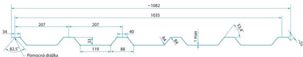
EVROtrapéz 35/N
